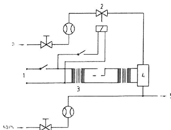
Figura 1 – Diagrama del dispositivo de ensayo de la eficacia del convertidor de NO 2
