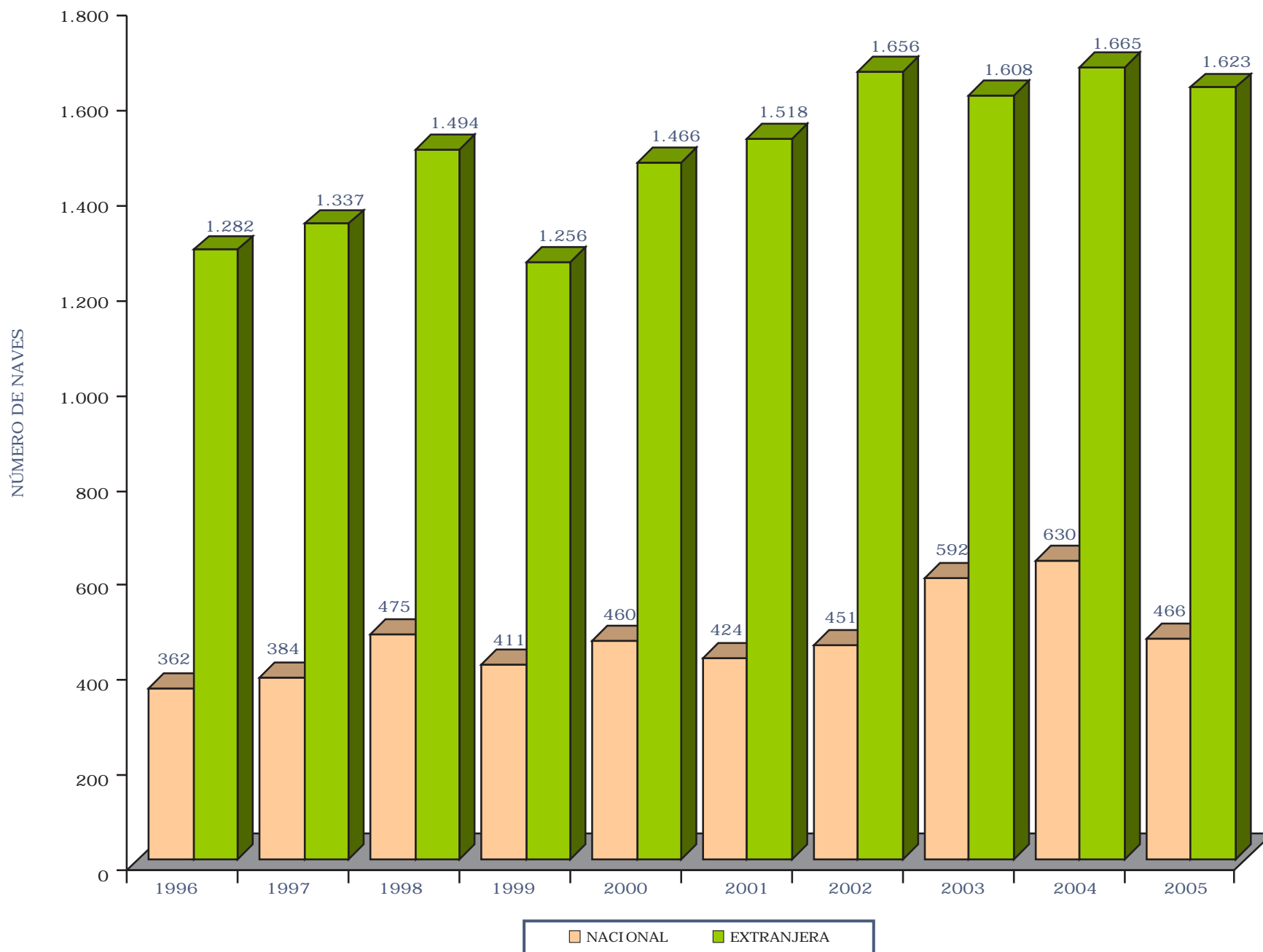
Gráfico 19: Tráfico Marítimo en el Estrecho de Magallanes. Años 1996-2005
