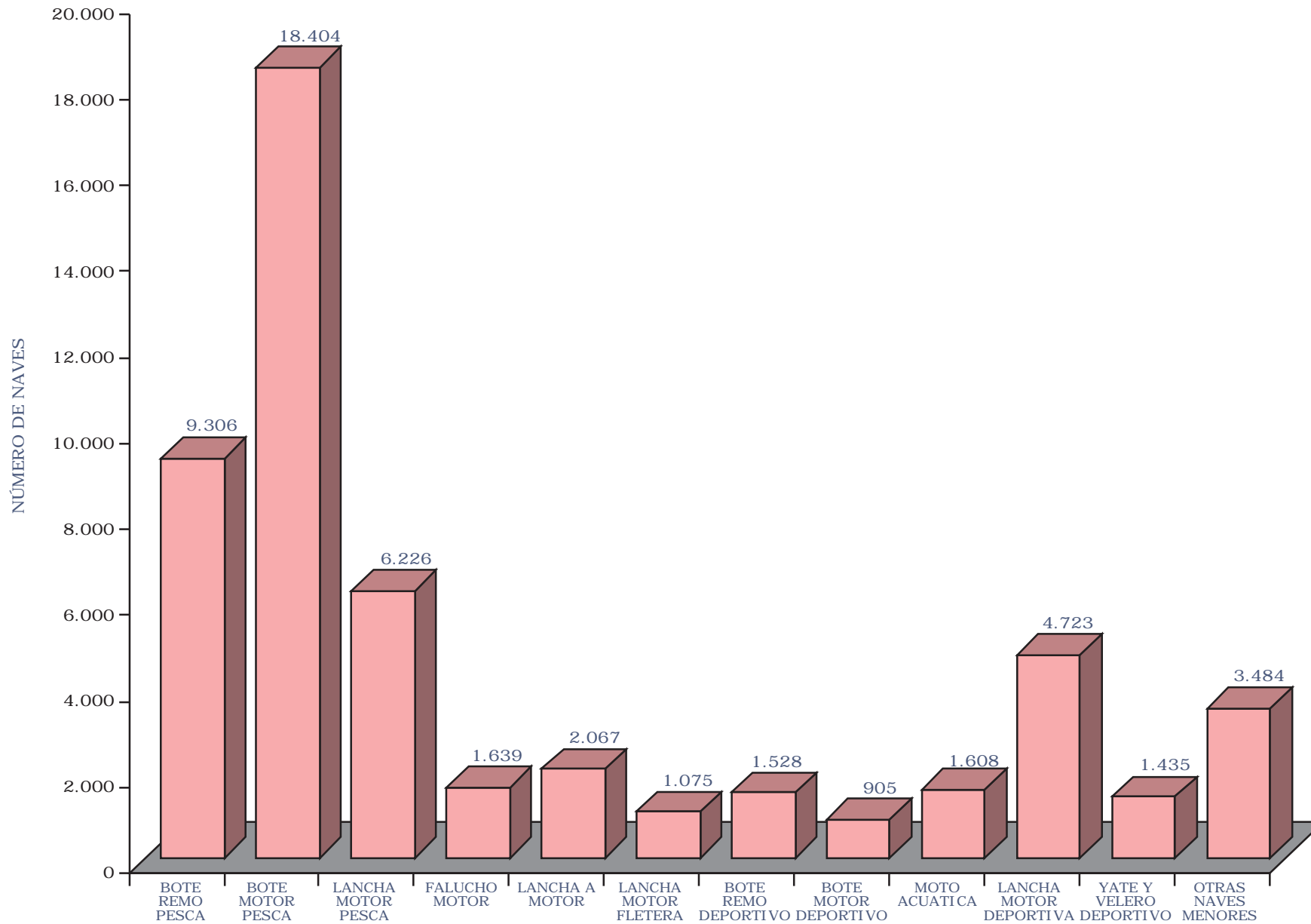
Gráfico 26: Naves Matriculadas Menores de 50 T.R.G. por Tipo, al 31 de Diciembre del 2005
