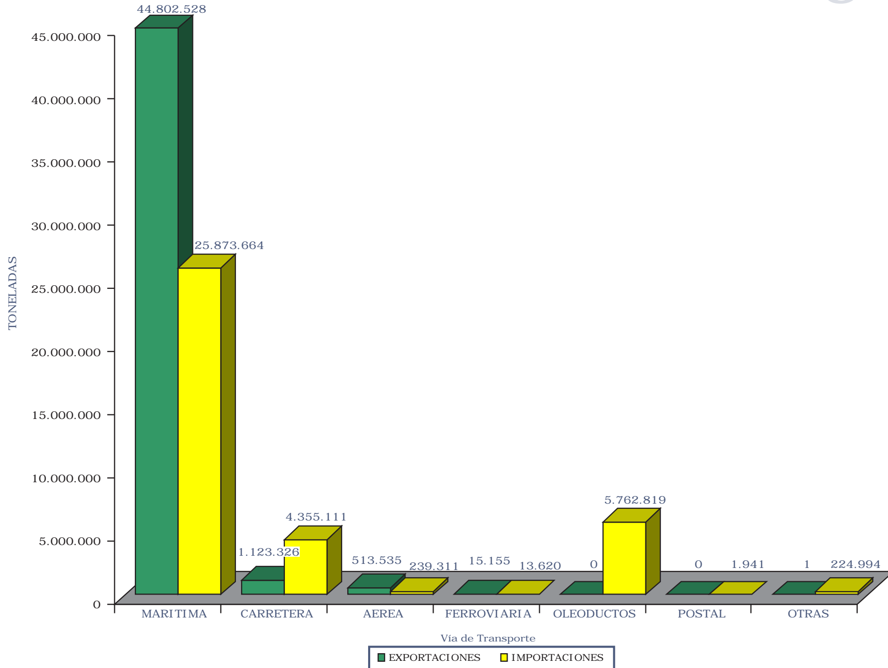
Gráfico 14: Tonelaje Movilizado en Comercio Exterior según Vía de Transporte. Año 2005
