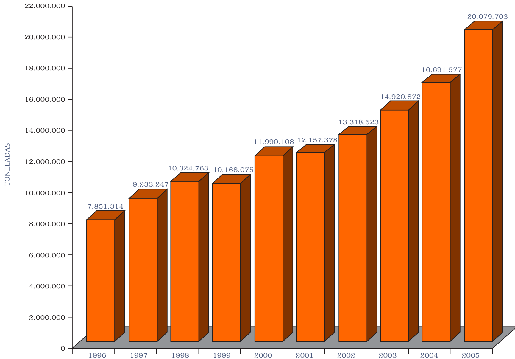
Gráfico 16: Tonelaje Movilizado en Contenedores. Años 1996-2005
