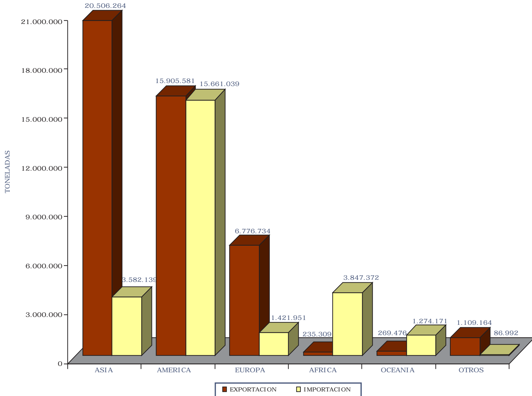
Gráfico 13: Tonelaje Exportado e Importado según Continente de Destino y Origen. Año 2005
