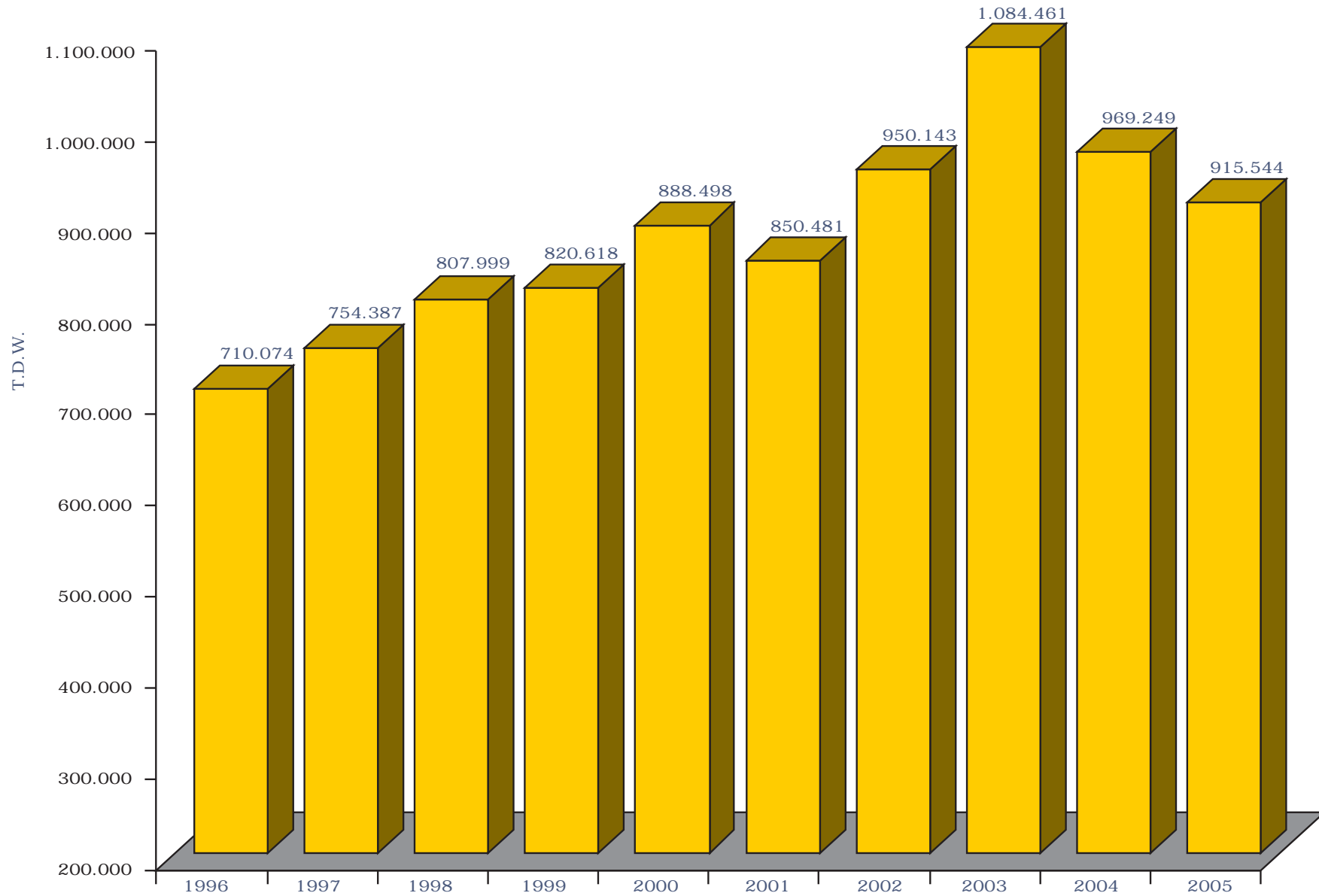
Gráfico 01: T.D.W. de la Flota de la Marina Mercante Nacional, desde 1996 a Diciembre del 2005
