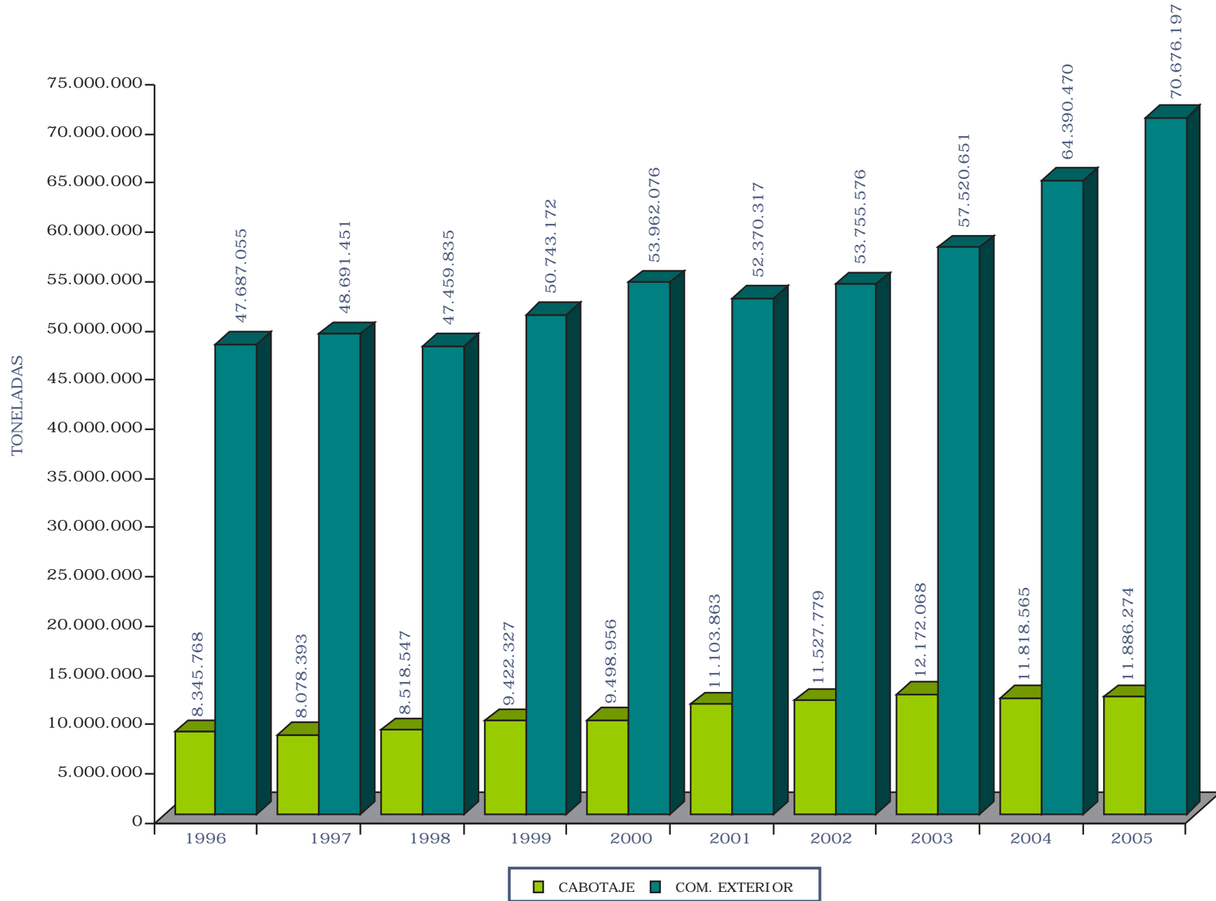
Gráfico 09: Tonelaje Movilizado por Servicio. Años 1996-2005
