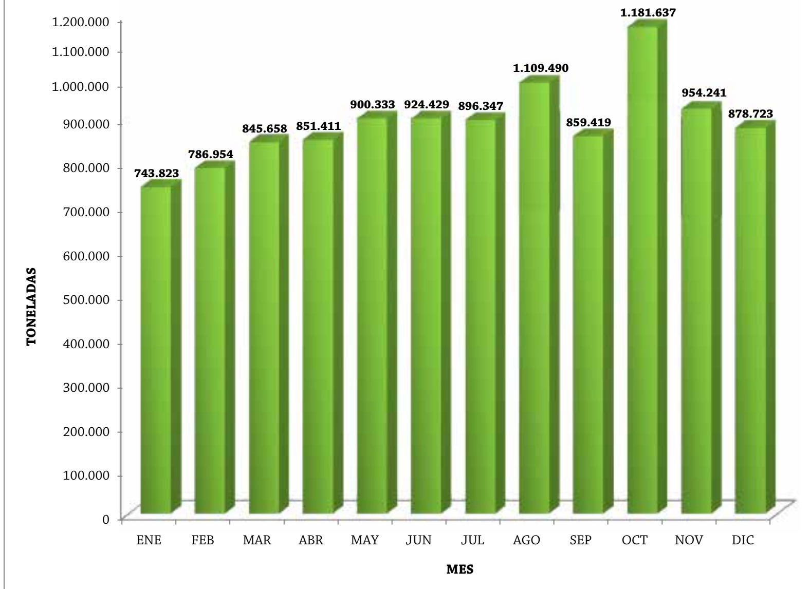
GRÁFICO 23: TONELAJE IMPORTADO MENSUAL DE CARGA TIPO GENERAL. AÑO 2012
