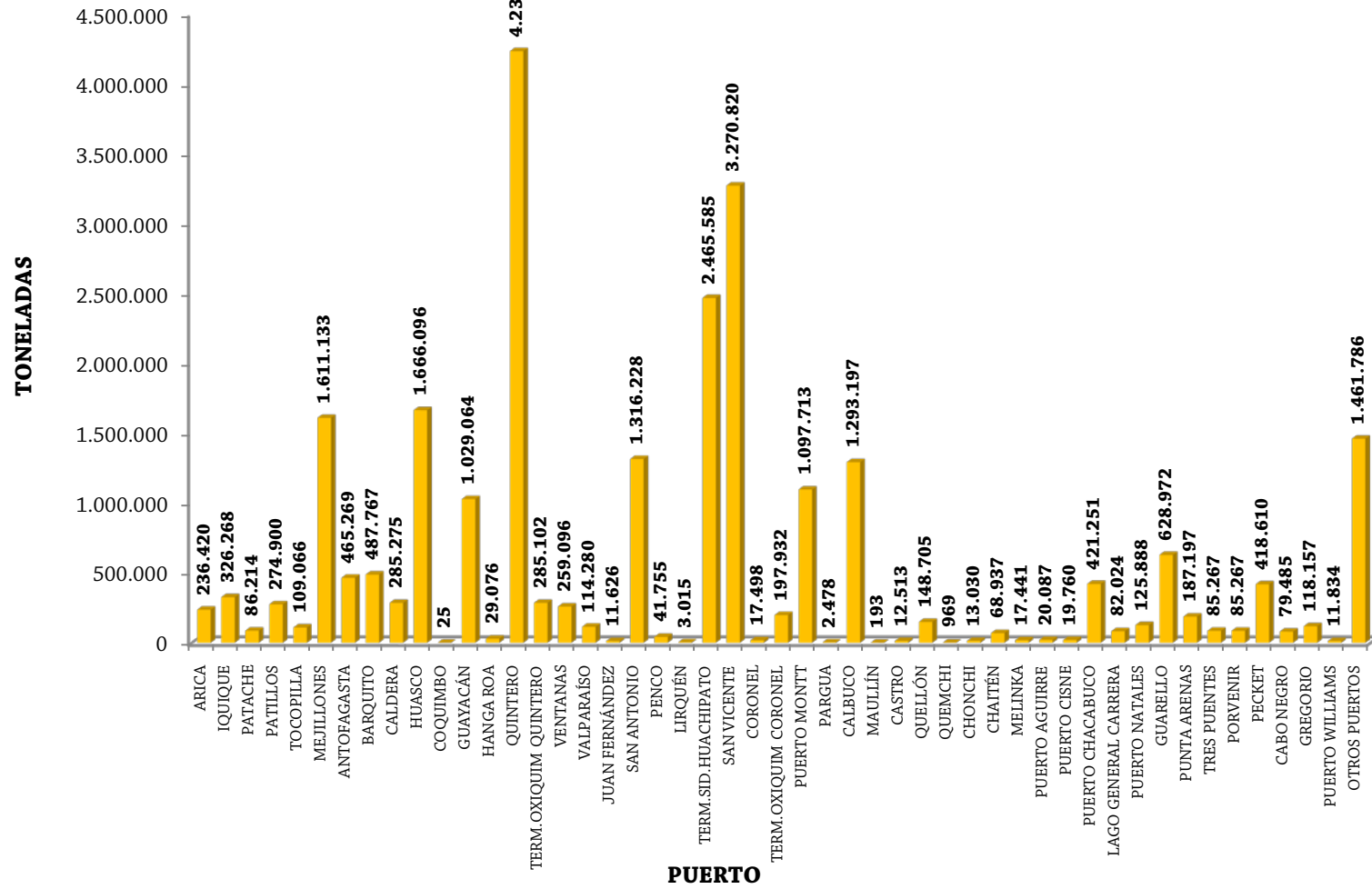
GRÁFICO 30: TONELAJE TOTAL MOVILIZADO EN CABOTAJE POR PUERTO. AÑO 2012
