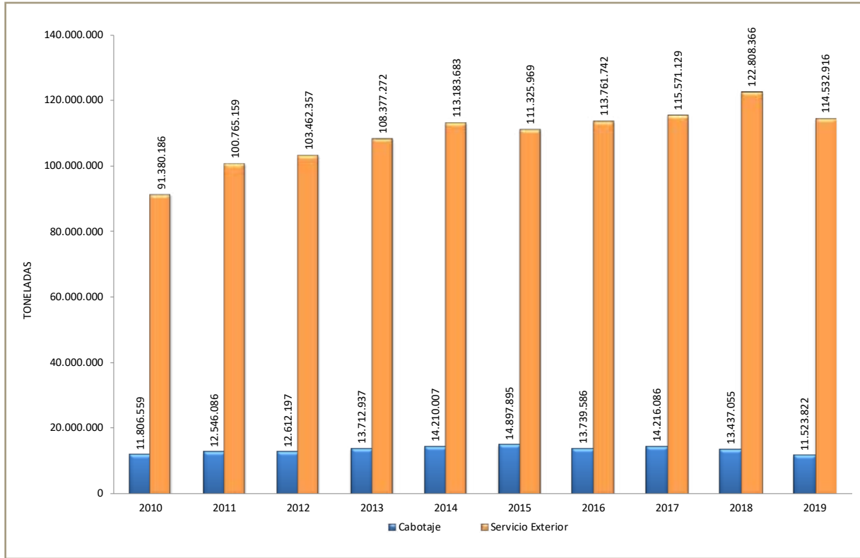
Gráfico 10: Tonelaje movilizado por servicio. Años 2010 - 2019
