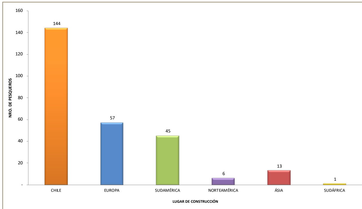
Gráfico 28: Distribución de los pesqueros de altamar según lugar de construcción Año 2019
