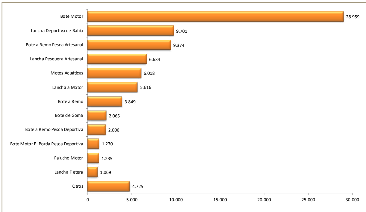
Gráfico 27: Número de naves matriculadas menores de 50 TRG. por tipo al 31 de diciembre del 2019
