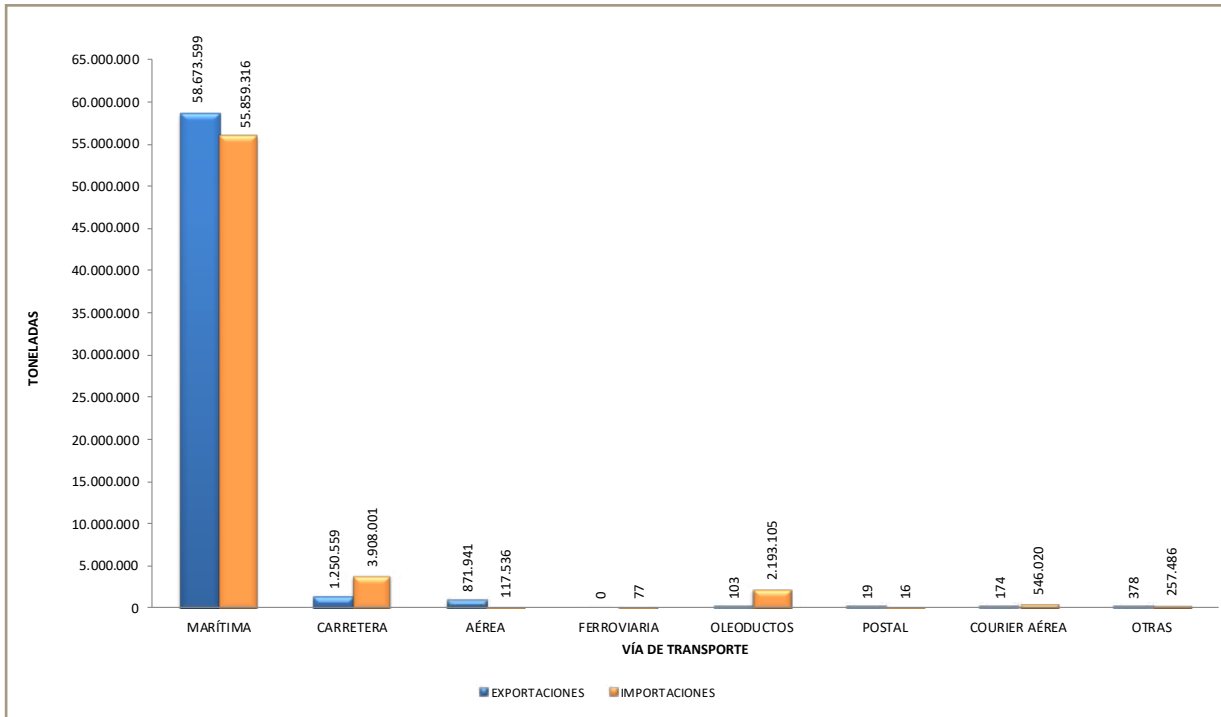
Gráfico 15: Tonelaje movilizado en comercio exterior según vía de transporte Año 2019
