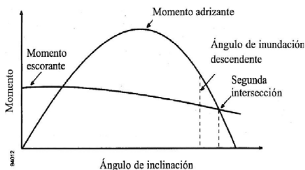
Figura 2.6-2: Curvas de momentos adrizantes y de momentos escorantes
