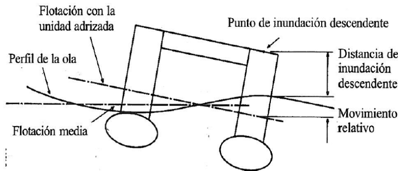
Figura 2.6-4: Definición de la distancia de inundación descendente y el movimiento relativo
