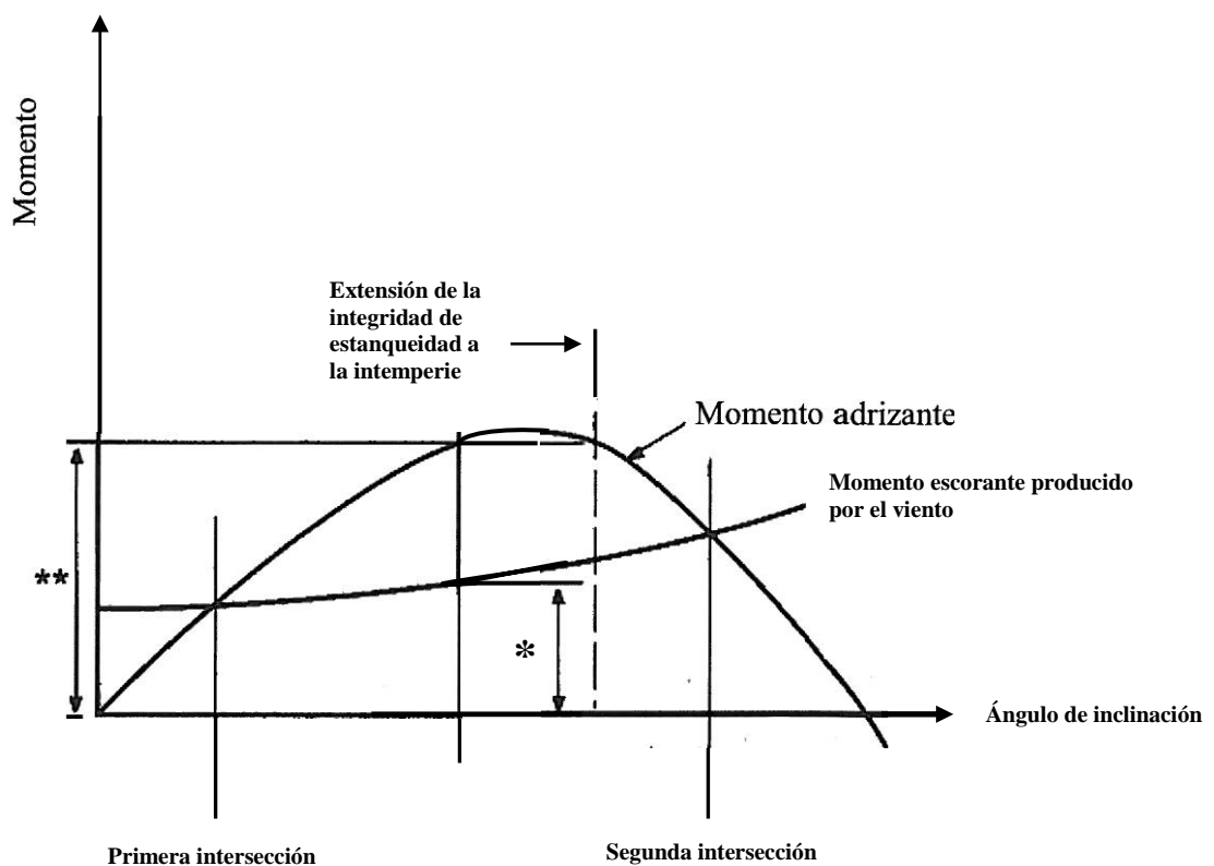
Figura 2.6-1: Curvas de momentos adrizantes y de momentos escorantes producidos por el viento
