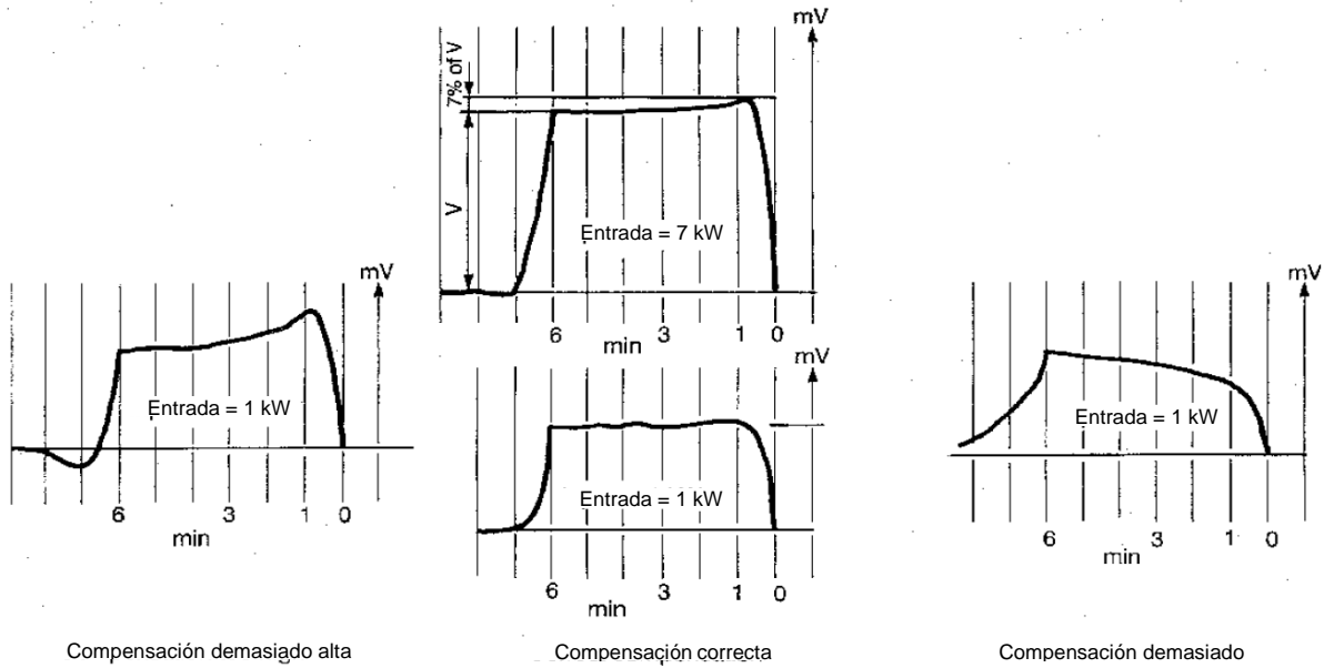
Figura 8 – Ejemplo de reacción de la señal de desprendimiento de calor ante un impulso térmico de onda cuadrada
