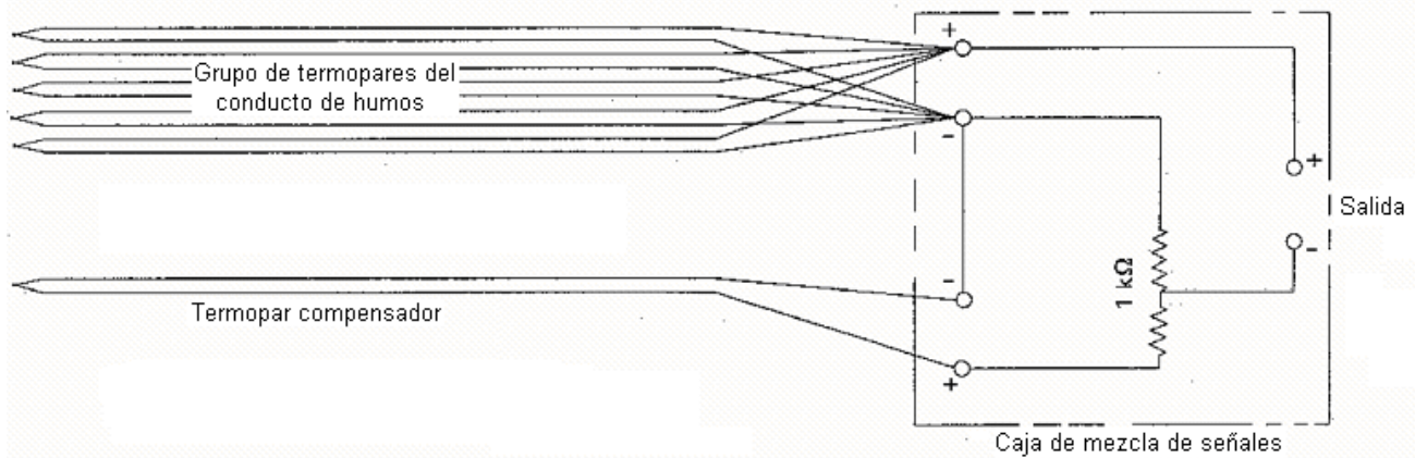
Figura 7 – Diagrama de un circuito de termopares
