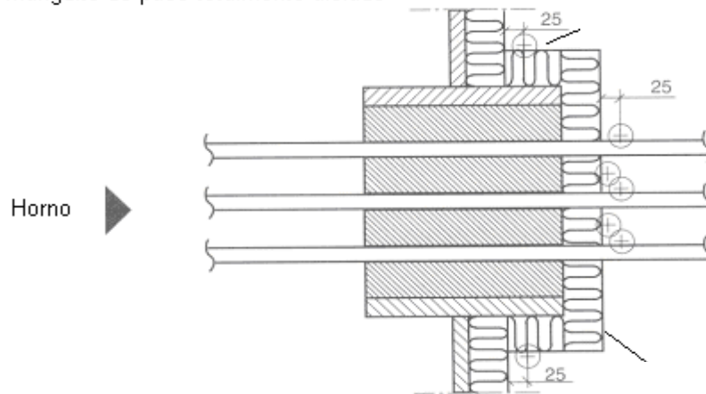
Manguito de paso totalmente aislado
