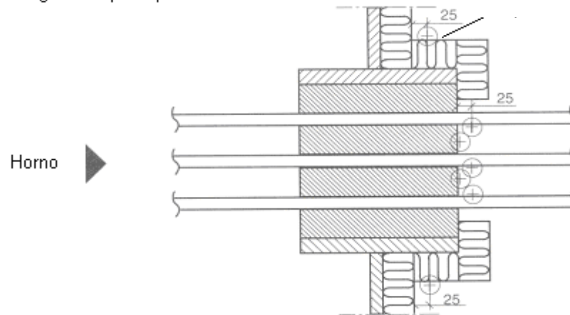
Manguito de paso parcialmente aislado
