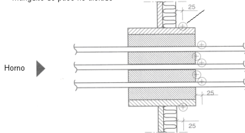
Manguito de paso no aislado
