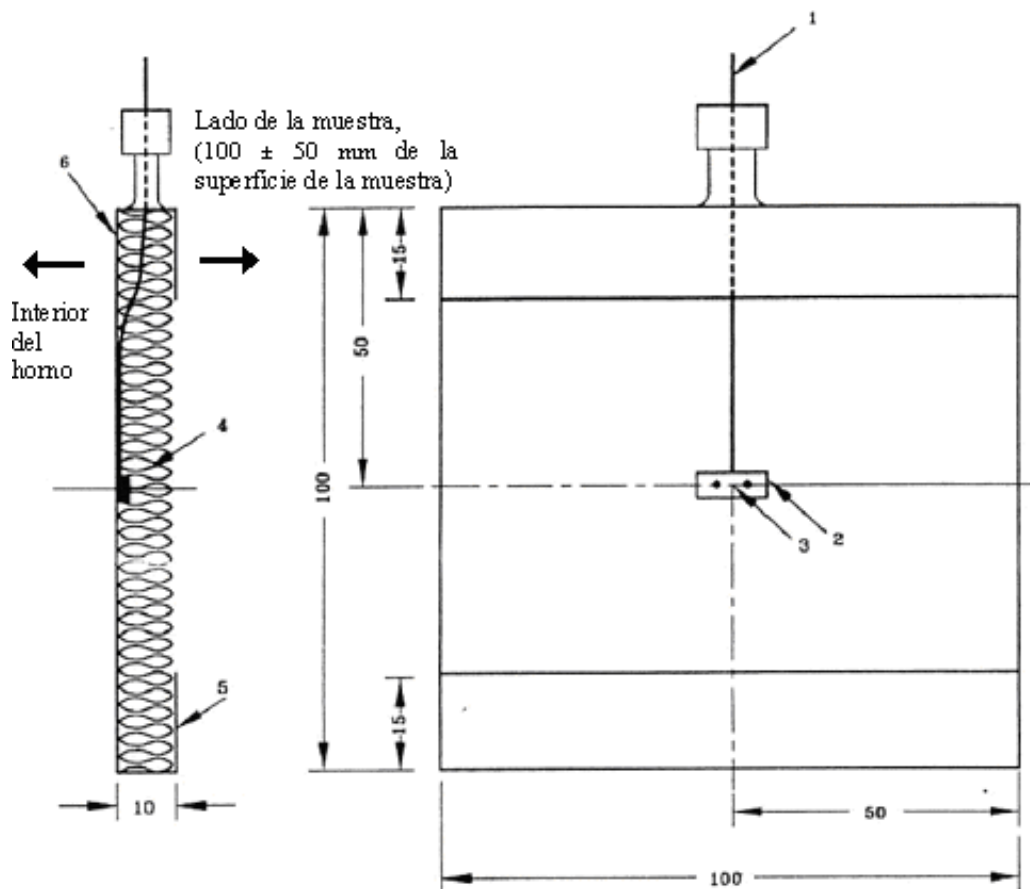
Figura 4 – Montaje de los termopares del horno
