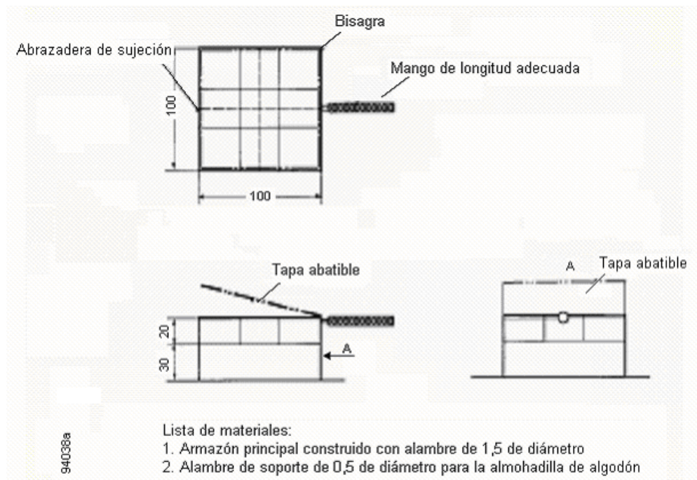
Figura 10 – Soporte de la almohadilla de algodón
