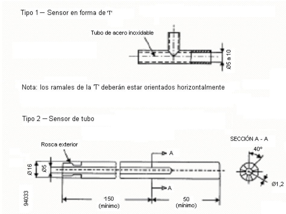
Figura 5 – Cabezas sensoras de presión
