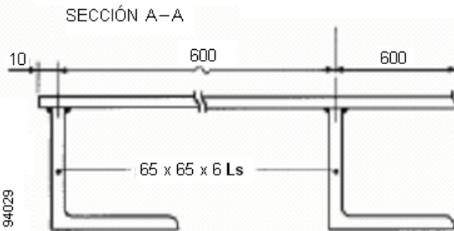
Figura 1 – Núcleo estructural de acero para mamparos de clase "A" y revestimientos de clase "B"
