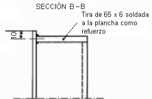
Figura 1 – Núcleo estructural de acero para mamparos de clase "A" y revestimientos de clase "B"
