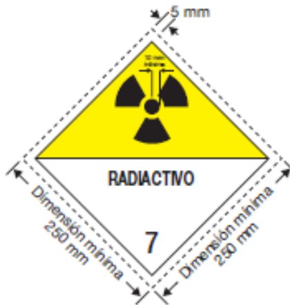
Rótulo para materiales radiactivos de la clase 7
