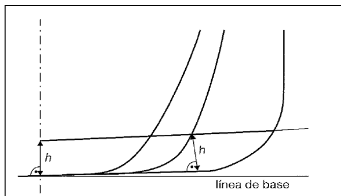
Figura 1: Límites de los tanques de combustible
