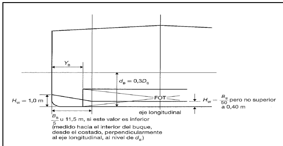
Figura 3: Dimensiones para el cálculo del escape mínimo de hidrocarburos
