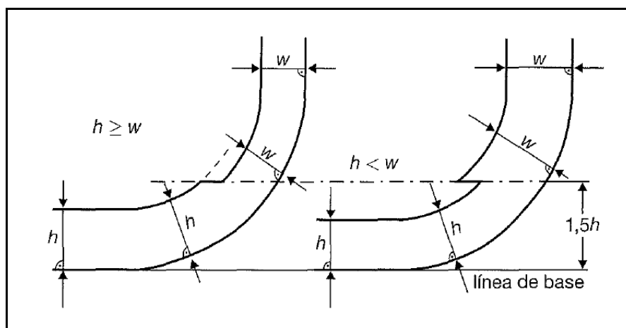
Figura 2: Límites de los tanques de combustible líquido
