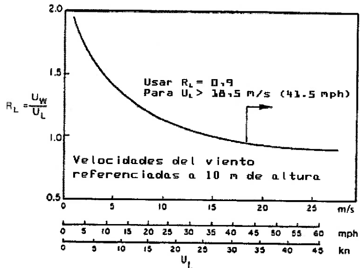
Figura 2: Relación entre la velocidad del viento sobre agua y sobre tierra.
