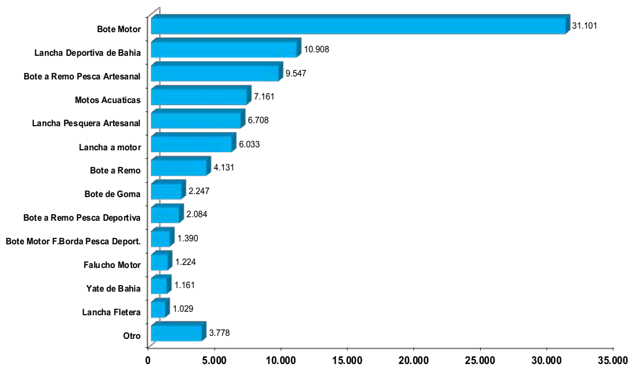
GRAFICO 27: NÚMERO DE NAVES MATRICULADAS MENORES DE 50 TRG. POR TIPO AL 31 DE DICIEMBRE DEL 2022
