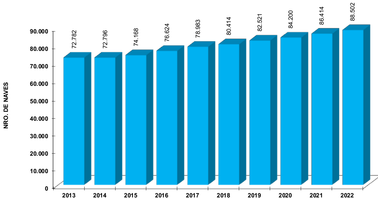
GRAFICO 26: NÚMERO DE NAVES MATRICULADAS MENORES DE 50 TRG AÑOS 2013 AL 2022
