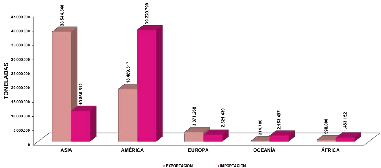
GRÁFICO 14: TONELAJE EXPORTADO E IMPORTADO SEGÚN CONTINENTE DESTINO Y ORIGEN AÑO 2022
